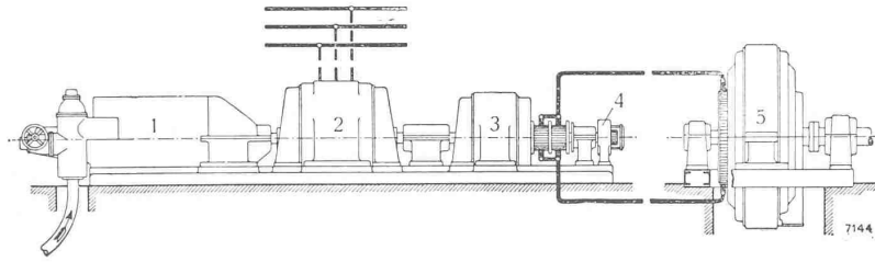
Abb. 13. Schema des Turbo-Fördersystems.
