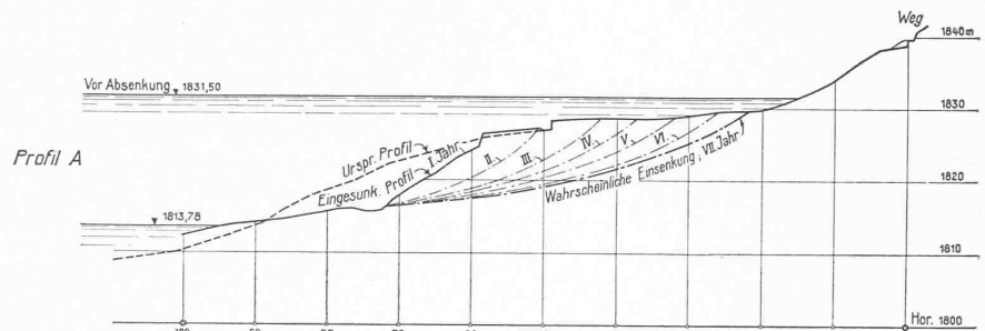
Ufer-Abbruchung am Ritomsee (ergänzte Abb. 3 von Seite 52). — Masstab 1 : 1000.
