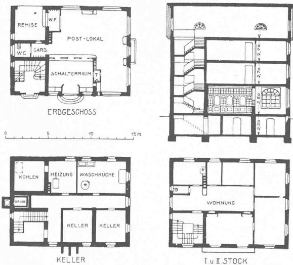
II. Preis. Entwurf Nr. 1. — Grundrisse und Schnitt 1:400.
