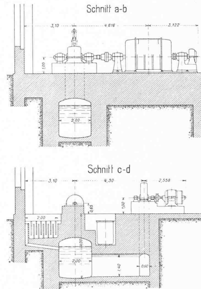
Die Wasserkraft-Anlage am Lac d'Oô in den französischen Pyrenäen.
