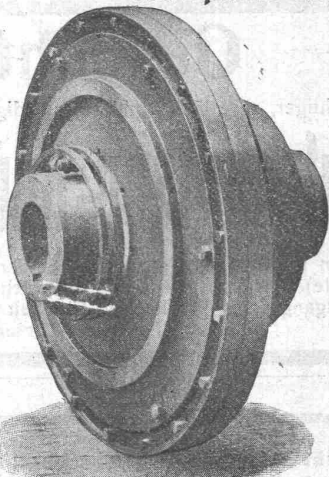
Elektromagnetische Reibungskupplung Patent.
