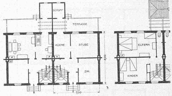
Grundrisse zu Typ B.
