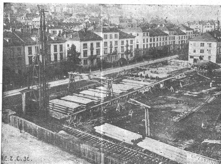
Postgebäude St. Gallen. Fundierung mit Eisenbetonpfählen, System Züblin.
