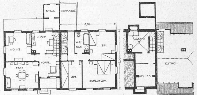
Bebauungsplan 1:3000. — Grundrisse des Dreizimmer- (ob.n), Vierzimmer- (links) und Fünzimmer-Hauses (rechts). — 1:300.
