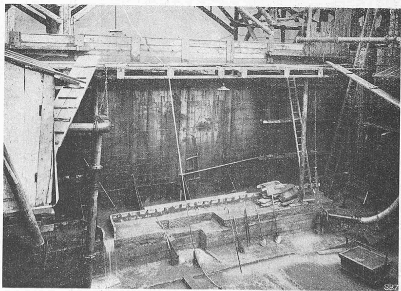
Abb. 17. Öffnung 5. Untere provisorische Abschlusswand, Schwelle noch unverkleidet (8. XII. 1915).
