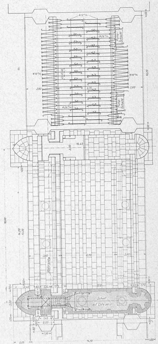
Abb. 12. Grundriss und Armierung der Wehrschwelle und Pfeilerschnitt.
