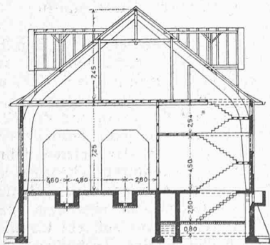
Abb. 8. Querschnitt. — Masstab 1 : 400.
