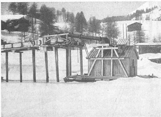
Abb. 1. Schwimmende Pumpstation im Davoser-See. April 1919. (Das im Winter vom Eis umschlossene Kanalgelüst ist bereits frei.)
