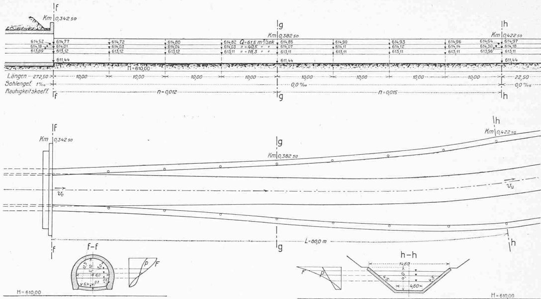
Abb. 2. Profil-Erweiterung — Masstab 1: 600.
