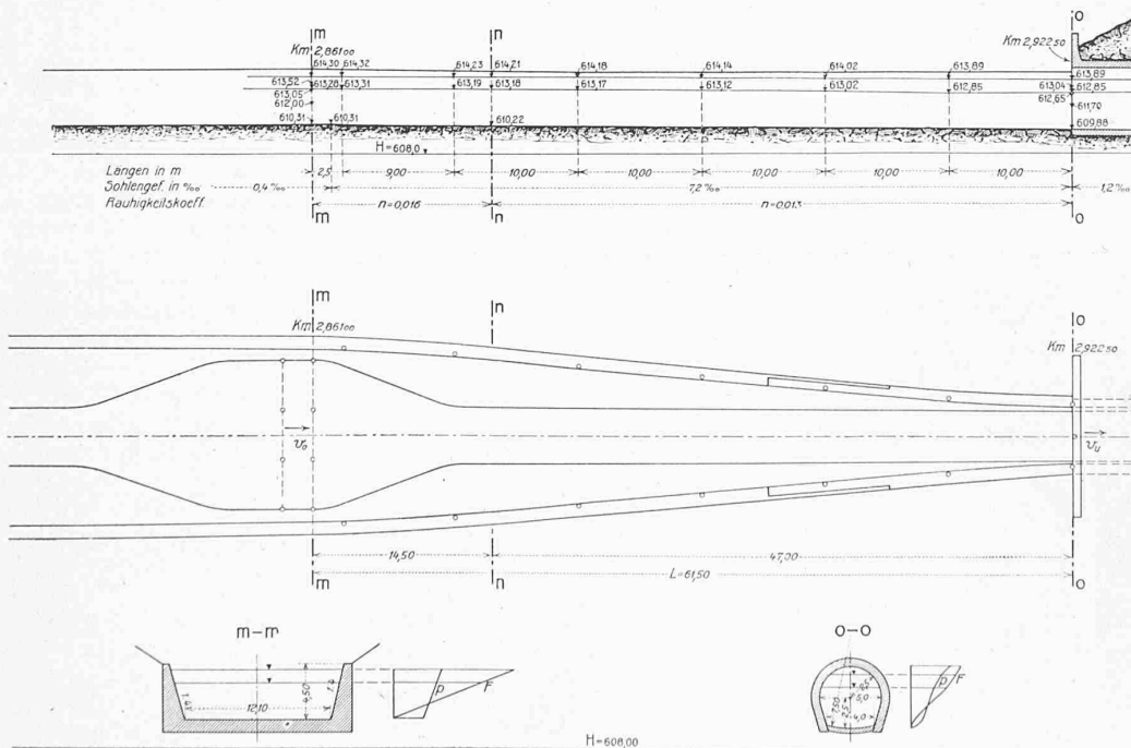
Abb. 4. Profil-Verengung. — Masstab 1: 600.
