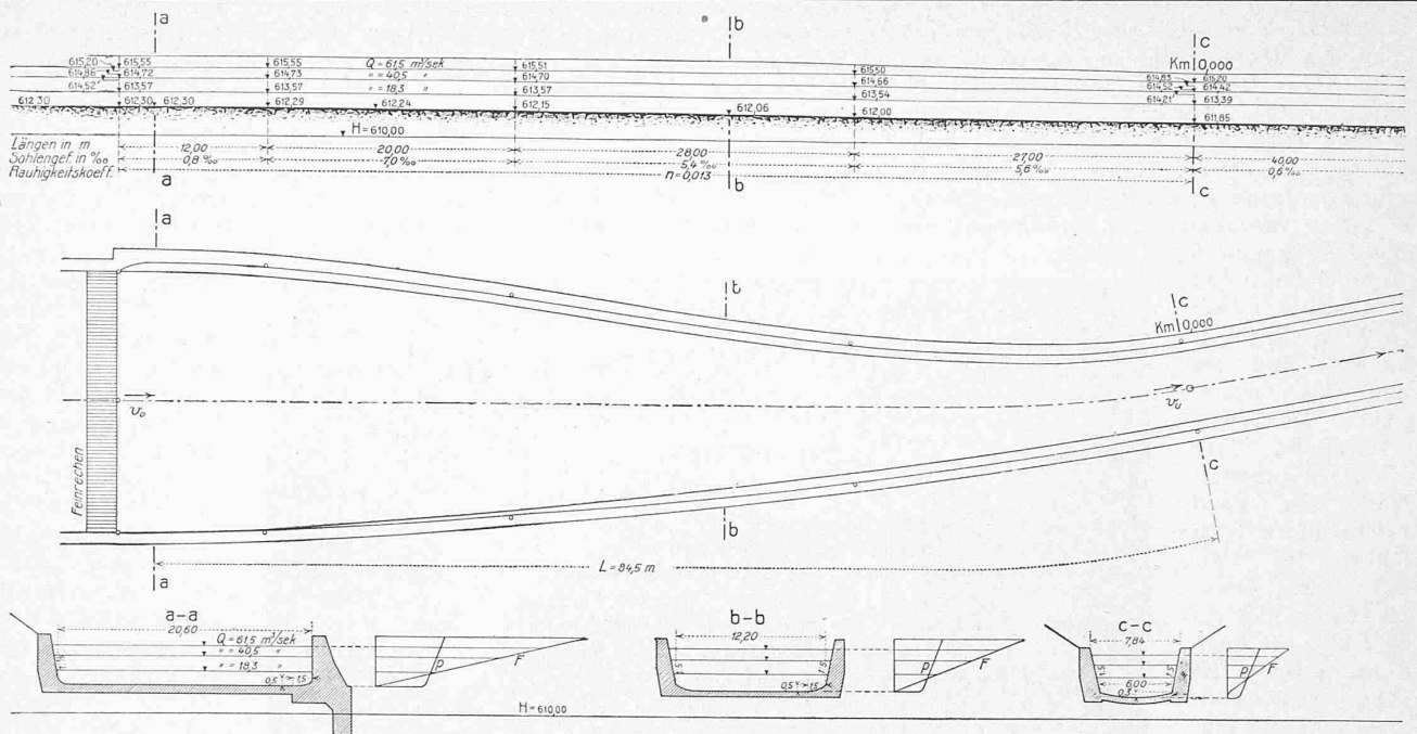
Abb. 1. Profil-Verengung. — Masstab 1:600.
