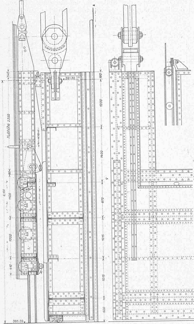
Abb. 34. Dichtungsfugen von der Oberwasserseite (Stellung I) vor Einschrauben der federnden Dichtungsbleche; rechts die Stauwand der obren Schütze.
