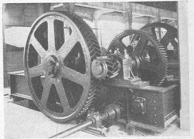
Abb. 36. Antrieb der Kettenachsen für die Gall'schen Ketten.
