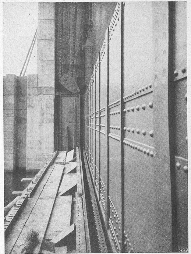
Abb. 34. Dichtungsfugen von der Oberwasserseite (Stellung I) vor Einschrauben der federnden Dichtungsbleche; rechts die Stauwand der obren Schütze.
