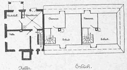
Fünfstück-Einfamilienhäuser Typ C
