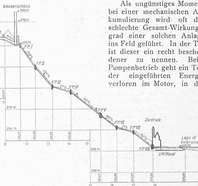
Abb. 2. Längenprofil der Druckleitung. — Längen 1 : 10 000, Höhen 1 : 2500. Querprofile des Druckstollens, 1 : 250.
