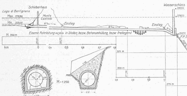
Abb. 2. Längenprofil der Druckleitung. — Längen 1 : 10 000, Höhen 1 : 2500. Querprofile des Druckstollens, 1 : 250.
