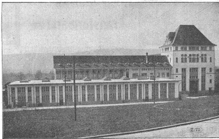
Schaltheus des Kraftwerkes Olten-Gösgen, erbaut 1915/17.
