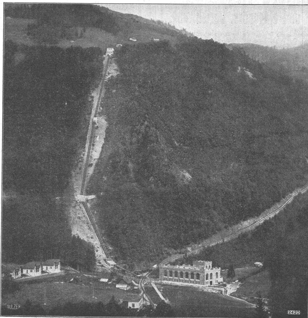
Hochdruckrohrleitungen des Elektrizitätswerkes Obermaif-Engelberg der Stadt Luzern
