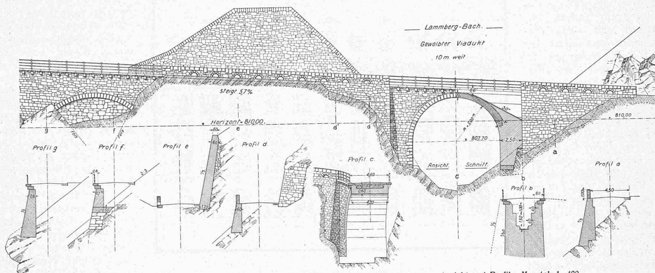
Abb. 10. Lehnbau zwischen Km. 1,35 (rechts) und 1,43 (links) in der Lammenschlucht. — Ansicht und Profile, Masstab 1:400.
