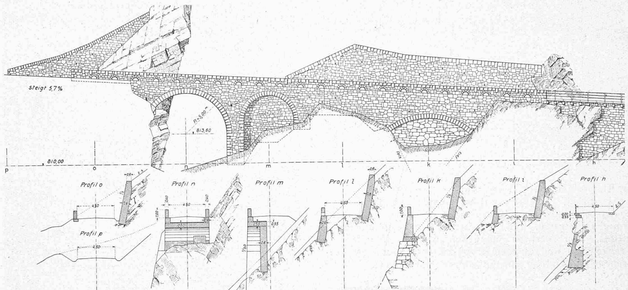
Abb. 11. Lehnbau zwischen Km. 1,43 (rechts) und 1,51 (links) in der Lammschlucht. — Ansicht und Profile, Masstab 1 : 400.
