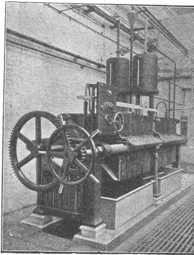
Apparat zur Herstellung von 6,5 m 3 H und 3,25 m 3 O pro Stunde.
