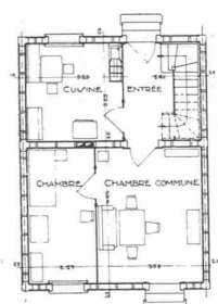
PLAN DU REZ-DE-CHAUSSEE
