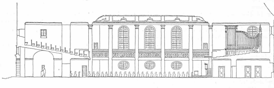
III. Preis, Entwurf Nr. 7. — Längsschnitt 1:375.
