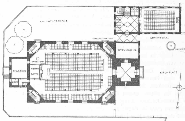
III. Preis, Entwurf Nr. 7. — Arch. Friedrich Hess, von Arbon, in Charlottenburg. — Grundrisse 1:750 und Innenansicht.
