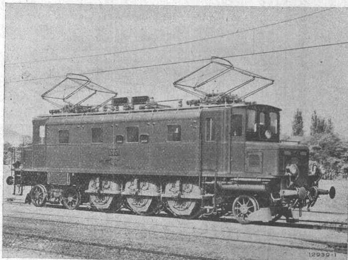
Einphasen-Schnellzugslokomotive mit Einzel-Achsantrieb Type 2-C-1 für die Schweizerischen Bundesbahnen, 3 x 700 PS, 1000 Volt Fahrdradhtspannung, 16 \frac{2}{3} Per/sec, max. Geschwindigkeit 60 bis 90 km/h.
