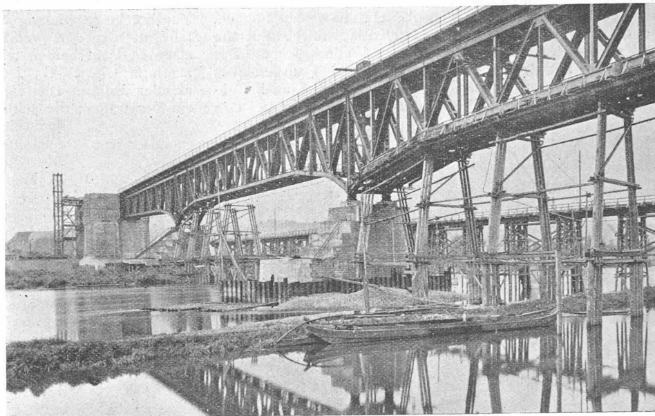
Abb. 7. Brücke über die Maas bei Visé. (Mittelöffnung von 93,00 m mit zwei Seitenöffnungen von je 75,50 m Weite.) Dahinter die Hilfsbrücke für den Erdtransport.
