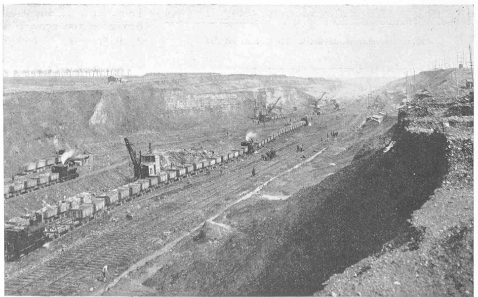
Abb. 9. Vom Bau der Hauptbahn Tongern-Aachen. — Grosse Einschnitt bei Visé, Km. 19 bis 20,3.
