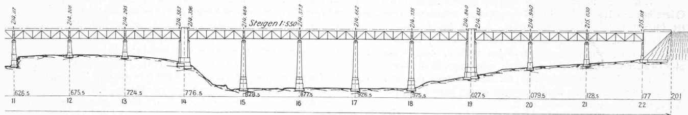
Abb. 13. Vom Bau der Hauptbahn Tongern-Aachen. — Brücke über das Geulthal, östliche Hälfte. — Masstab etwa 1:3000.
