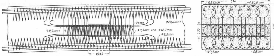
Abb. 4. Längsschnitt und Querschnitt durch das provisorische Scheitelgelenk. — Masstab 1:35.
