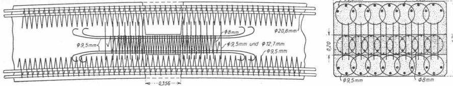
Abb. 4. Längsschnitt und Querschnitt durch das provisorische Scheitelgelenk. — Masstab 1:35.
