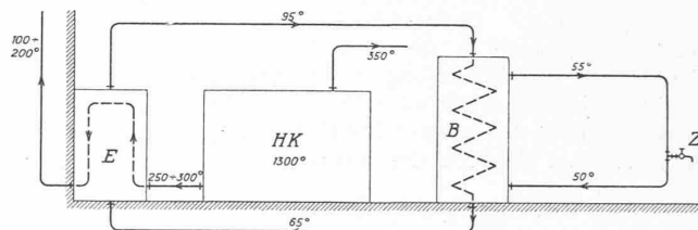
Abb. 5. Ofen mit Abhitze-Kessel. Abb. 6. Hochdruck-Kessel mit Economiser. Abb. 7. Economiser, zum Betrieb einer Warmwasserversorgung dienend. LEGENDE zu Abb. 5 bis 7: O = Einsatz-, Glüh-, Härte- und Schmelz-Ofen; A = Abhitze-Kessel zur Dampf- oder Heisswasser-Bereitung; HK = Hochdruck-Dampfkessel; E = Economiser, in Abb. 6 in üblicher Weise als Speisewasser-Vorwärmer, in Abb. 7 zur Heizung eines Boilers dienend; Z = Zapfstelle.
