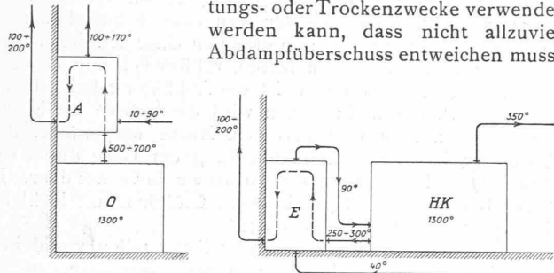
Abb. 5. Ofen mit Abhitze-Kessel. Abb. 6. Hochdruck-Kessel mit Economiser. Abb. 7. Economiser, zum Betrieb einer Warmwasserversorgung dienend. LEGENDE zu Abb. 5 bis 7: O = Einsatz-, Glüh-, Härte- und Schmelz-Ofen; A = Abhitze-Kessel zur Dampf- oder Heisswasser-Bereitung; HK = Hochdruck-Dampfkessel; E = Economiser, in Abb. 6 in üblicher Weise als Speisewasser-Vorwärmer, in Abb. 7 zur Heizung eines Boilers dienend; Z = Zapfstelle.
