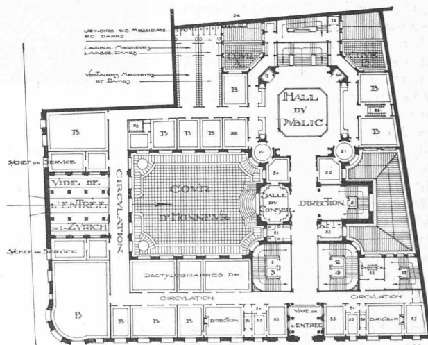
Abb. 18. Obergeschoss-Grundriss. — 1:800.
