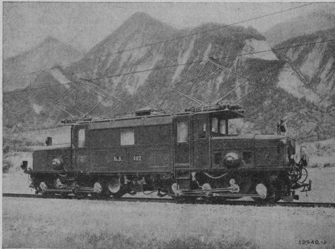
Einphasenstrom-Lokomotive, Type C-C für die Rhätische Bahn 2 × 600 PS, 10000 Volt, Fahrdrachtspannung 16 2 / 3 Per/sec, Geschwindigkeit 30 bis 45 km/h, Spurweite 1 m.
