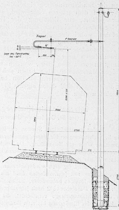
Abb. 13. Abzüge für Innenkurven mit Radien unter 300 m. — 1:100.
