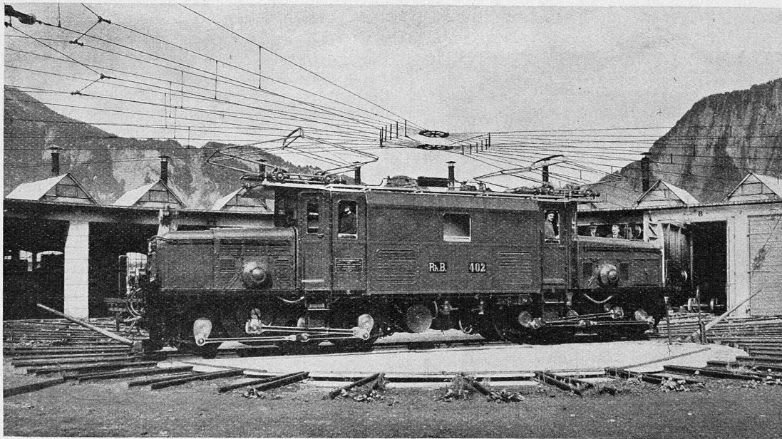
Abb. 10. Fahrleitungen, als Schutzstrecke geschaltet, über der Drehscheibe beim Lokomotivdepot Landquart.
