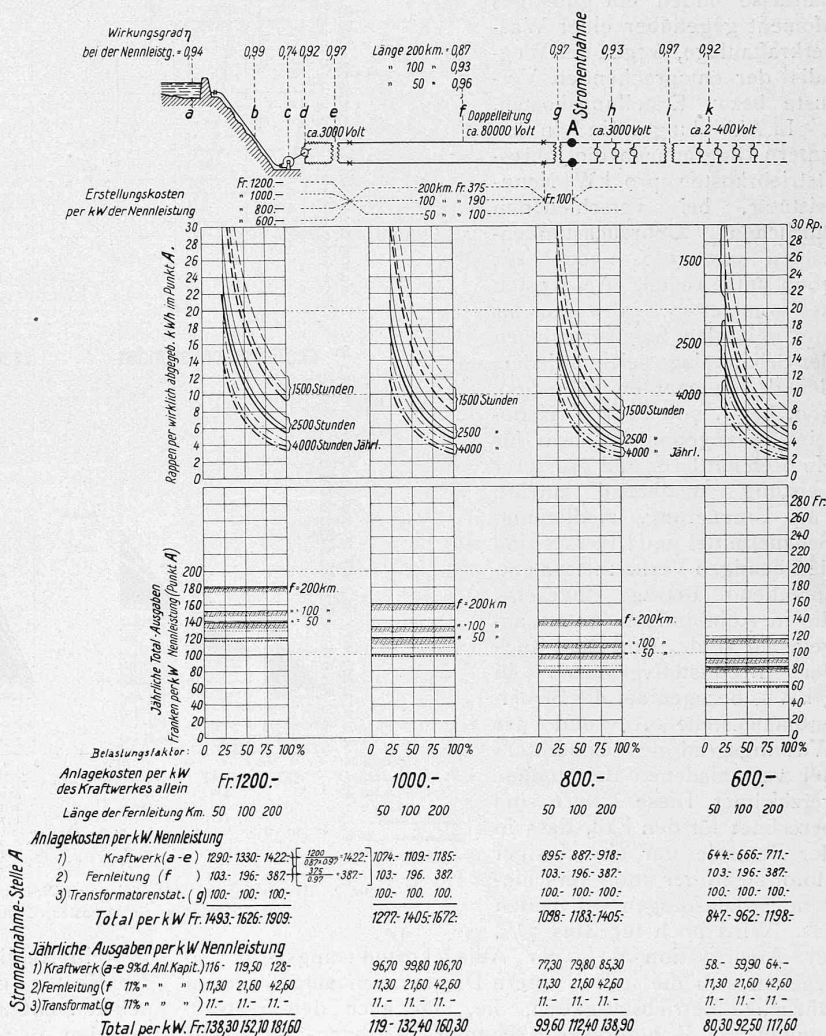
Abb. 1. Berechnung der kWh-Preise von Wasserkraft-Anlagen (Einphasenstrom 3000 V) für verschiedene Anlagekosten, Gebrauchstundenzahlen, Belastungsfaktoren und Fernleitungslängen.
