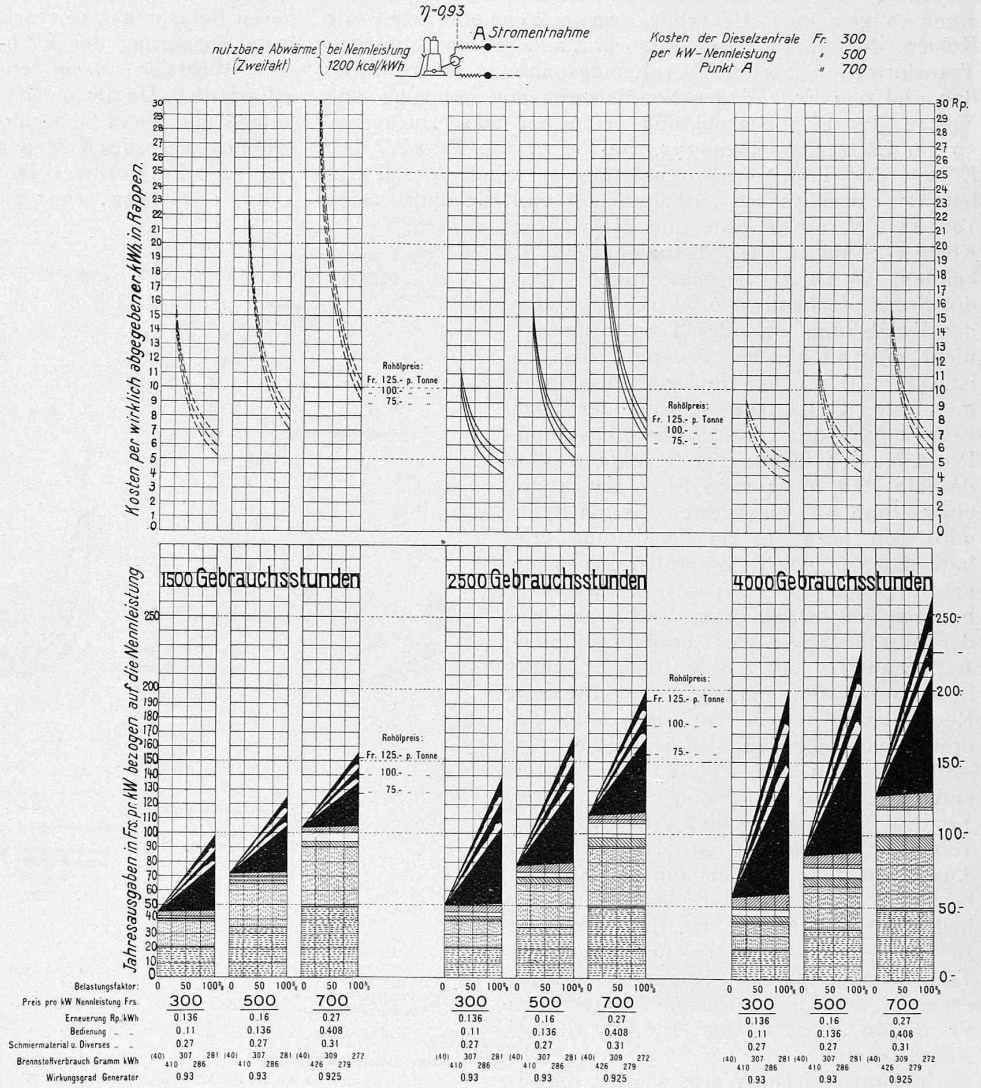
Abb. 2. Berechnung der kWh-Preise von Dieselmotor-Zentralen (beliebige Stromart und Spannung) für verschiedene Anlagekosten, Gebrauchstundenzahlen und Rohöl-Preise.
