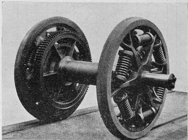
Abb. 15. Federnde Verbindung zwischen Hohlwelle und Triebzahnrad.
