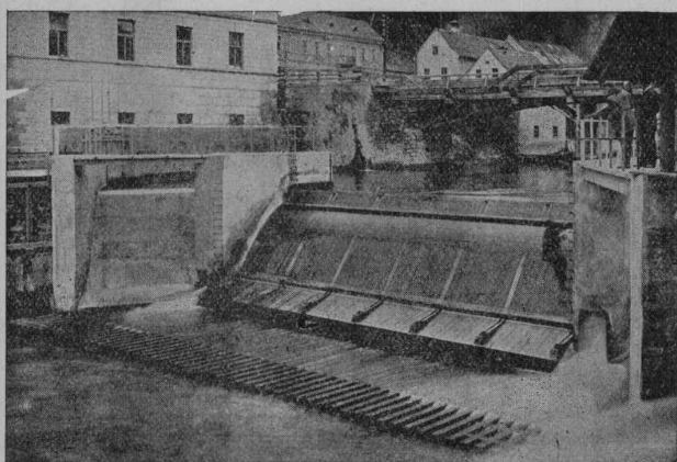
Dachwehr in der Müz der Kabelwerke Felten & Guilleaume, Brucka. d. Mur.
