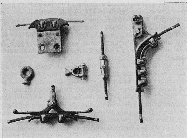
Abb. 13. Verbindungsmuffe, Abspann-, Stütz- und Hängesklammern.
