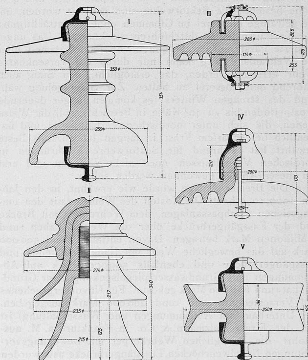
Abb. 14. Für die Albula-Leitung verwendete Isolatoren-Typen. I Hänge-Isolator Typ Motor, II Stütz-Isolator Typ Rosenthal, III Hänge- und Abspann-Isolator Typ Jeffery-Dewilt, IV Hänge- und Abspann-Isolator Typ Rosenthal, V Abspann-Isolator Typ Motor.
