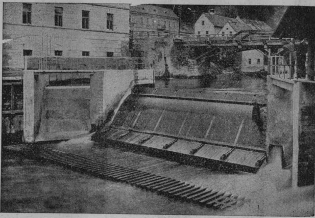
Dachwehr in der Mürz der Kabelwerke Felten & Guillaume, Bruck a. d. Mur.
