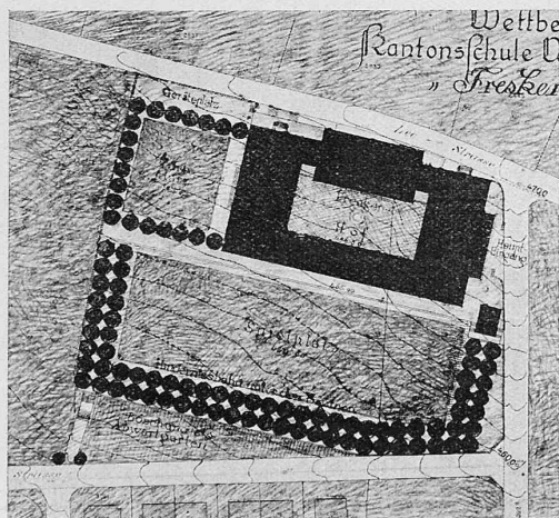
IV. Preis, Entwurf Nr. 53. — Architekten Vogelsanger &amp; Maurer, Rüschlikon. — Lageplan mit Variante, 1:2500.
