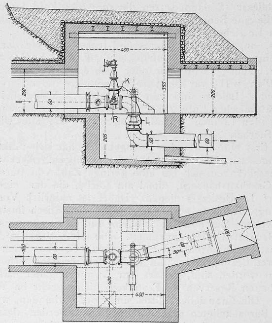
Abb. 11. Schieberhaus mit automatischem Ventil (L), 1:150, am untern Ende des 440 m langen Anstichstollens.
