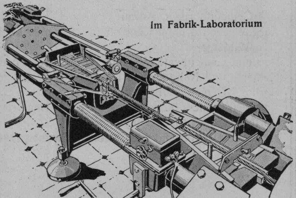
Drahtseil-Zerreiss-Versuch
