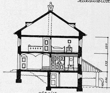
Schnitt
