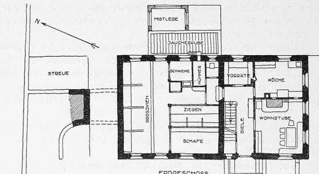
ERDGESCHOSS
