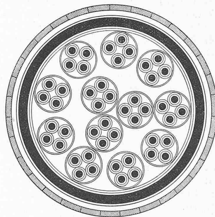
Abb. 2. Gotthard-Telephonkabel. — Querschnitt 1:1.
