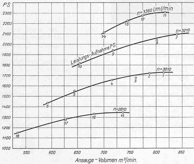
Abb. 14. Leistungsaufnahme des Hochofen-Turbogebläses bei mittlern p_1 = 0,983 at abs. und mittlern t_1 = 17,9^\circ\text{C} .
