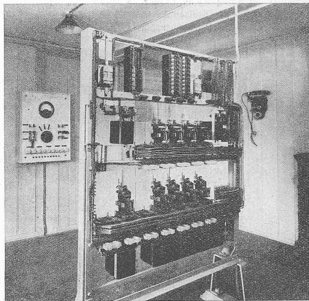
Abb. 3. Automatische Zentrale der Rh. B. in Landquart.
