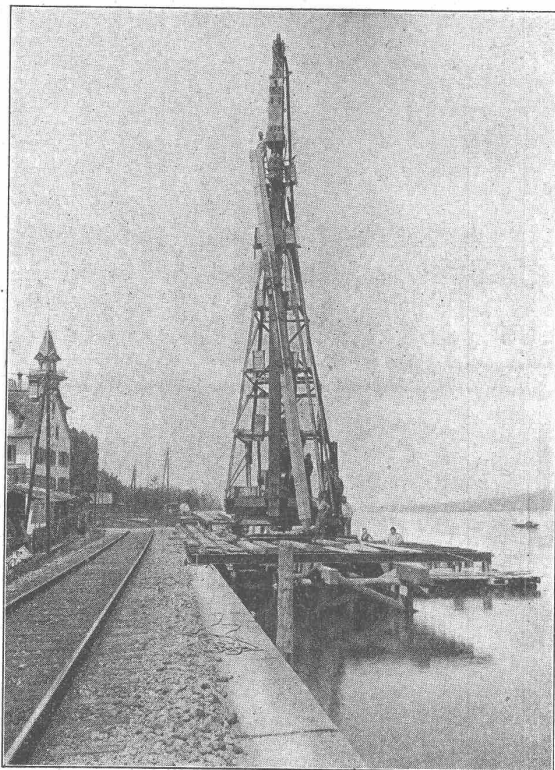
Fundierung einer Ufermauer in Wädenswil mit 22 m langen Eisenbetonpfählen System Züblin (z. Zt. im Bau)
