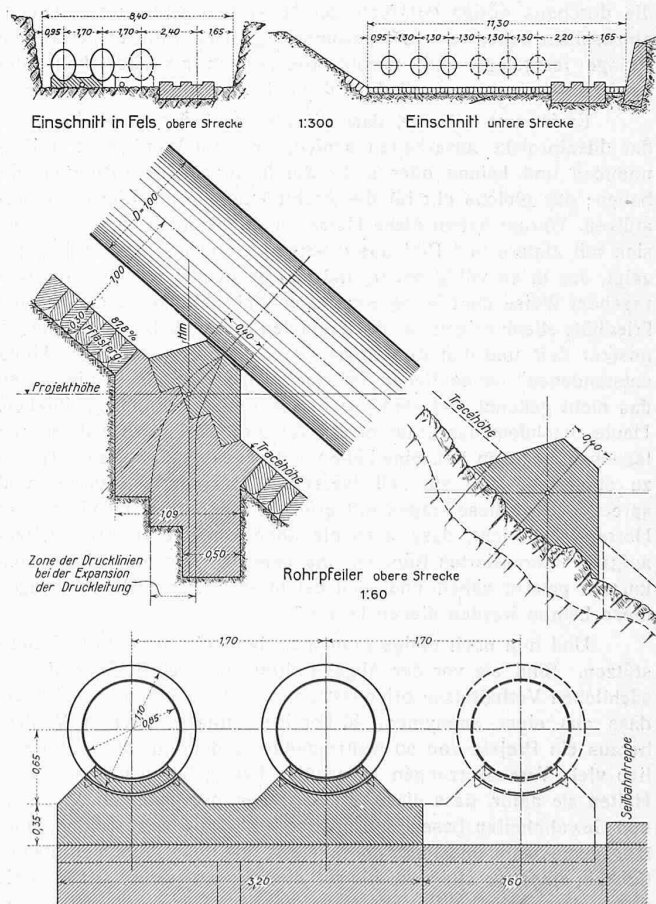
Abb. 25. Rohrbahnprofile in der oberen und in der unteren Strecke. — 1 : 300. Konstruktion der Rohrpfiler in der oberen Strecke. — 1 : 60.
