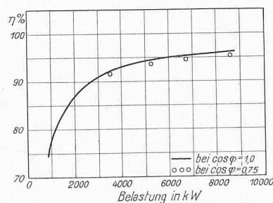
Abb. 63. Wirkungsgrade des Generators.
