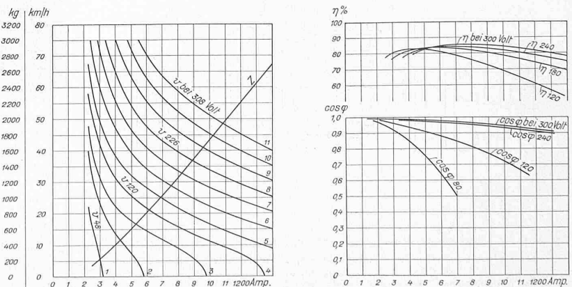
Abb. 9. Charakteristische Kurven der Triebmotoren von 200 PS Stundenleistung. Z = Zugkraft am Radumfang, v = Geschwindigkeit, \eta = Wirkungsgrad auf den R.-U. bezogen.
