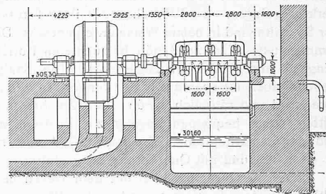
Abb. 1 bis 3. Grundriss des Maschinenraums des Schwarzenbachwerkes mit Ansicht der Gruppe I (JMV-Turbine) und Schnitt der EWC-Turbine — 1:300.
