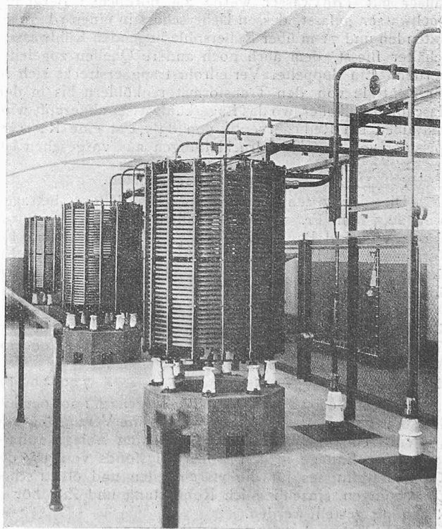
Abb. 90. Ueberstromschutz der Transformatoren.
