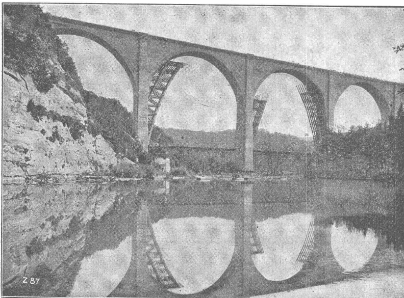
Pérollesbrücke in Fribourg (erbaut 1920—22).
