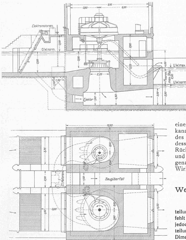
Abb. 8 bis 10. Moderne Konstruktions-Anlage. — Schnitte 1:20.
