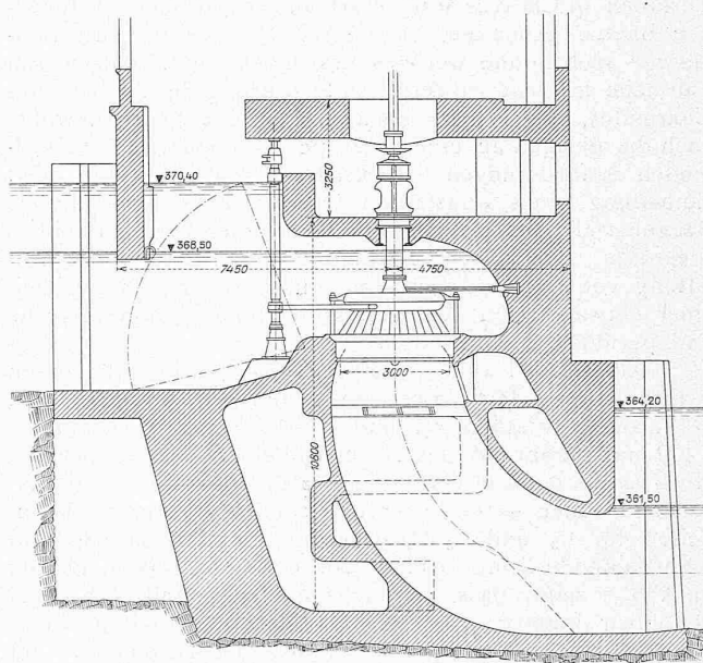
Abb. 4. Neue einfache Konusturbine.
